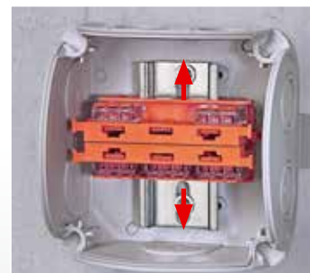
Клеммный блок может сдвигаться в обе стороны вдоль DIN-рейки.
